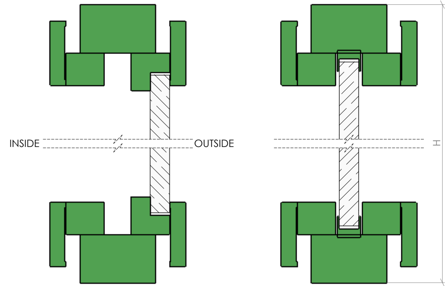
SECTION B-B SCALE 1 : 2
