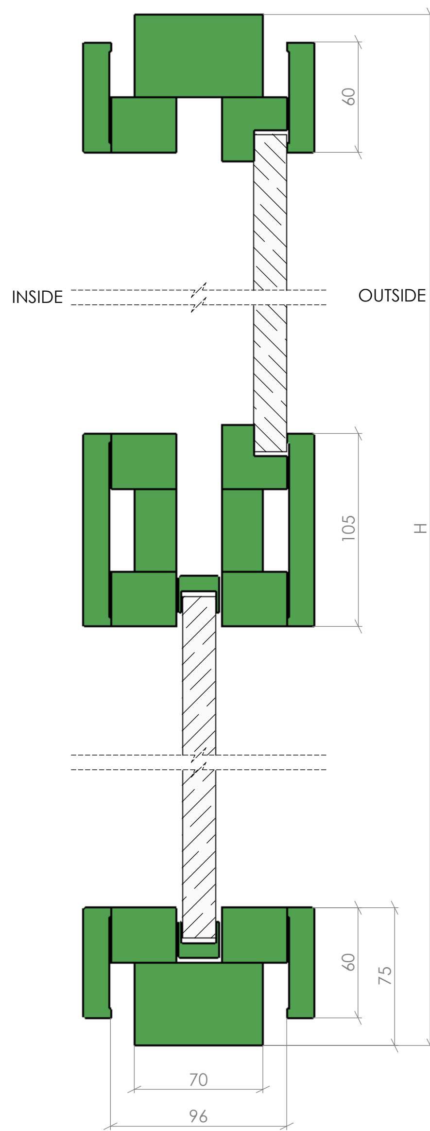
SECTION A-A SCALE 1 : 2
