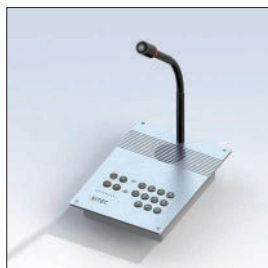
Infälld version Silver (130 x 190 x 34 mm) 111-08111
